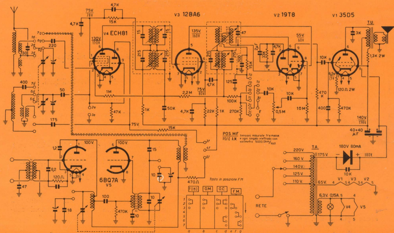
SCHEMA ELETTRICO FM/199
